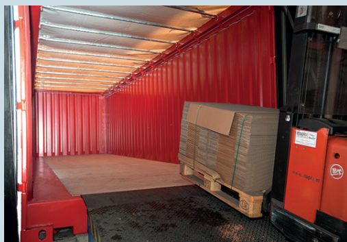
Be- und Entladung mit Stapler von hinten Loading and unloading with forklift truck from the rear
